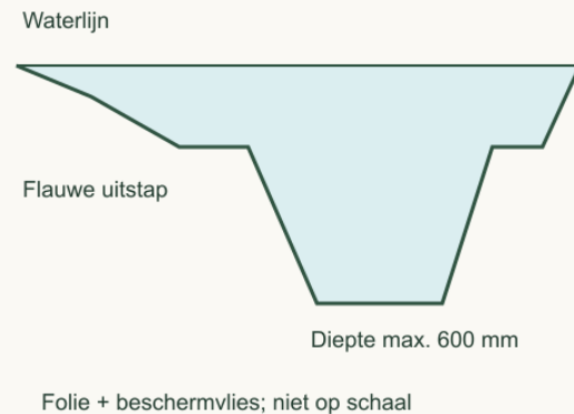
02 ZIJAAANZICHT / PRINCIPE
